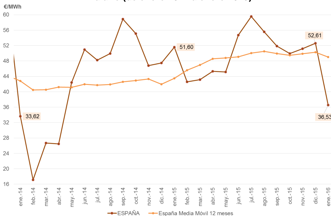
Gráfico 23. Precio medio mensual y media móvil anual del mercado diario (de enero 2014 a enero 2015)
