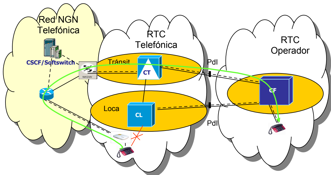
Servicio de interconexión de acceso ofrecido por Telefónica
