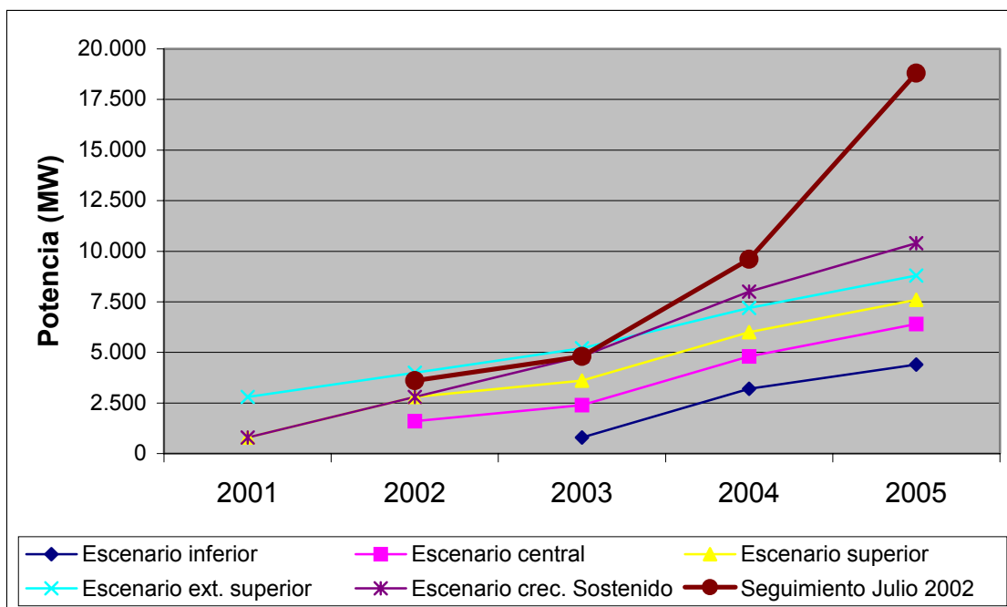
Figura 3.1 Escenarios de demanda de potencia punta contemplados en el Informe Marco y senda de incorporación de Ciclos Combinados según la información aportada por los promotores en el Proceso de Seguimiento de infraestructuras.
