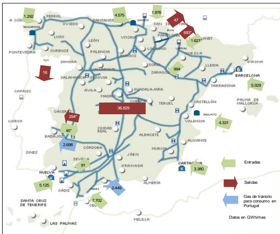
Figura 5. Entradas / salidas en la red de transporte.
