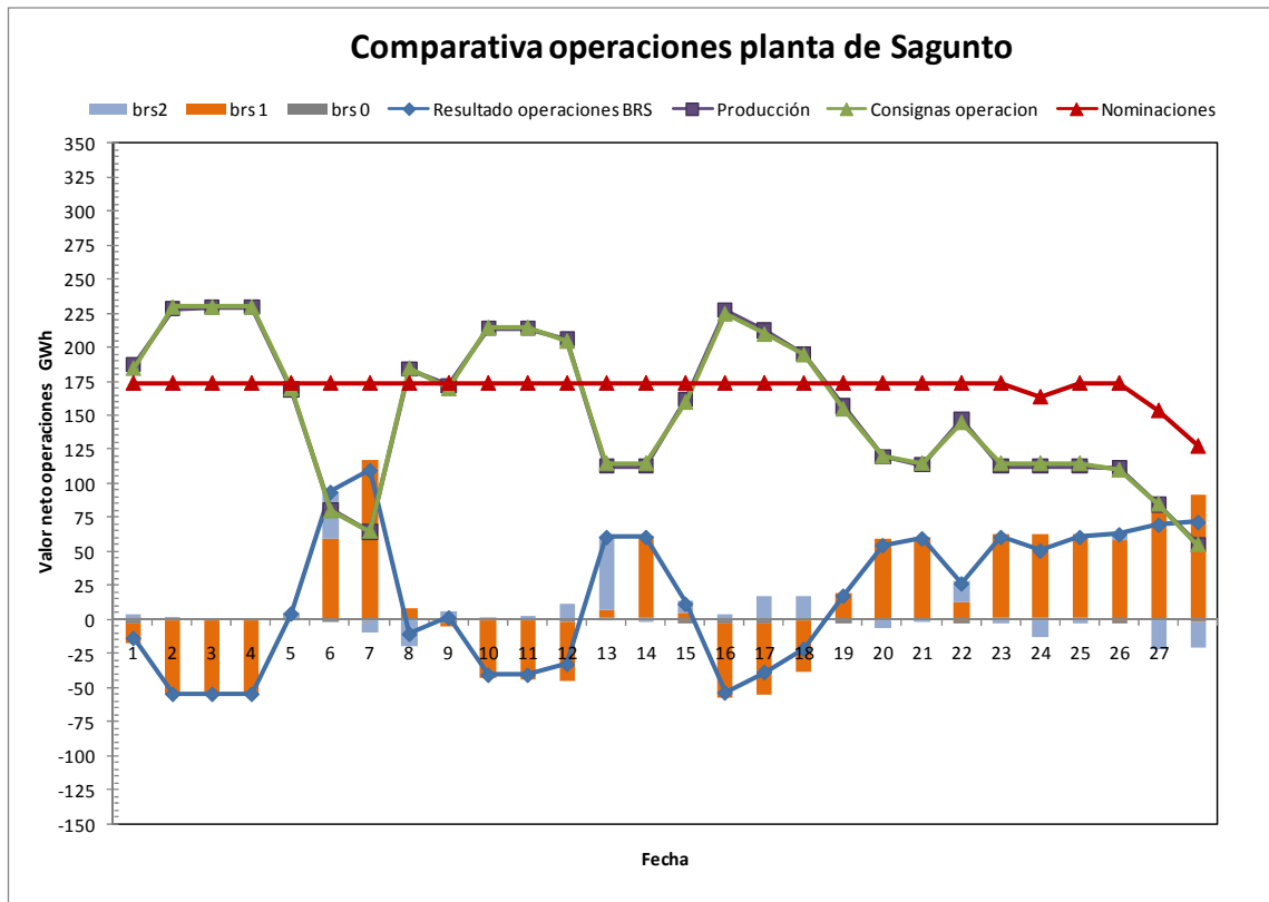
Figura 9. Comparativa consignas y operaciones BRS en Planta de Sagunto.
