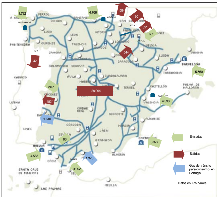
Figura 5. Entradas / salidas en la red de transporte.
