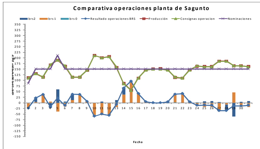
Figura 10. Comparativa consignas y operaciones BRS en Planta de Sagunto
