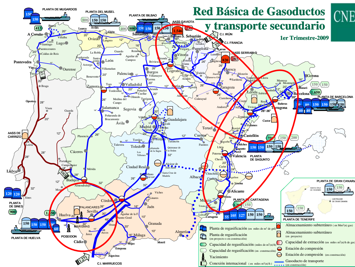
Gráfico 13: Red básica de gasoductos en el año 2008.
