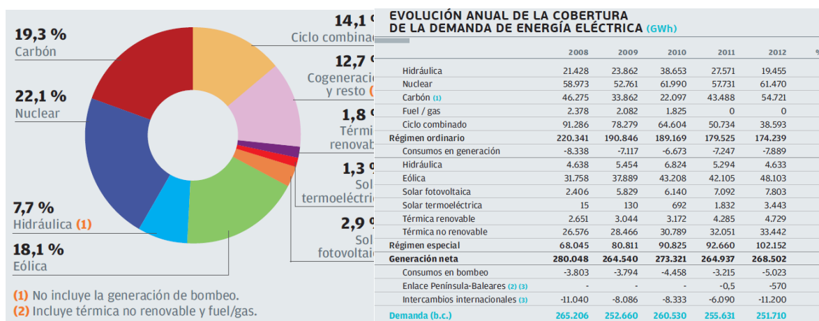
Gráfico 4. Estructura de generación neta acumulada 2012.
