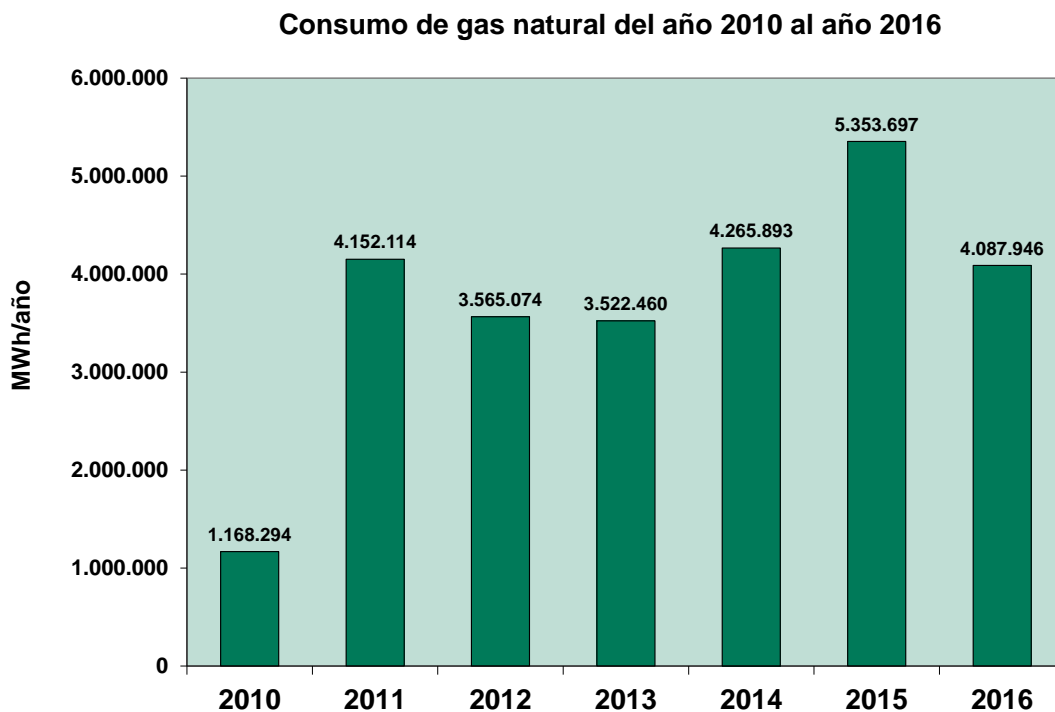
Gráfico 1. Consumo de gas natural en Baleares del año 2010 al año 2016.
