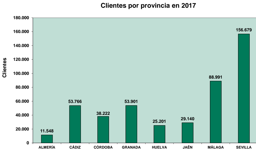
Figura 3. Número de clientes de gas natural en la Comunidad de Andalucía en el año 2017, por provincias.
