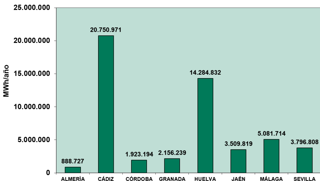
Figura 1. Consumo de gas natural en Andalucía en el año 2017, por provincias.
