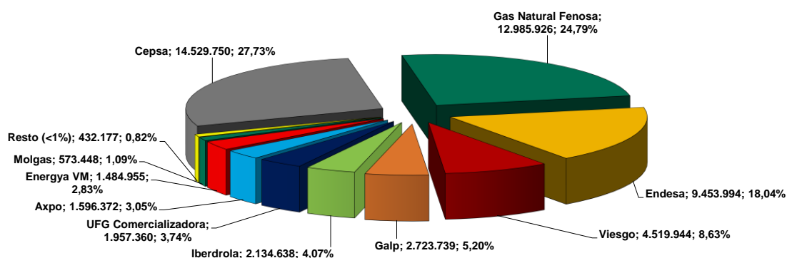
Figura 5. Cuotas de mercado por volumen de ventas de gas natural en la Comunidad de Andalucía en el año 2017.
