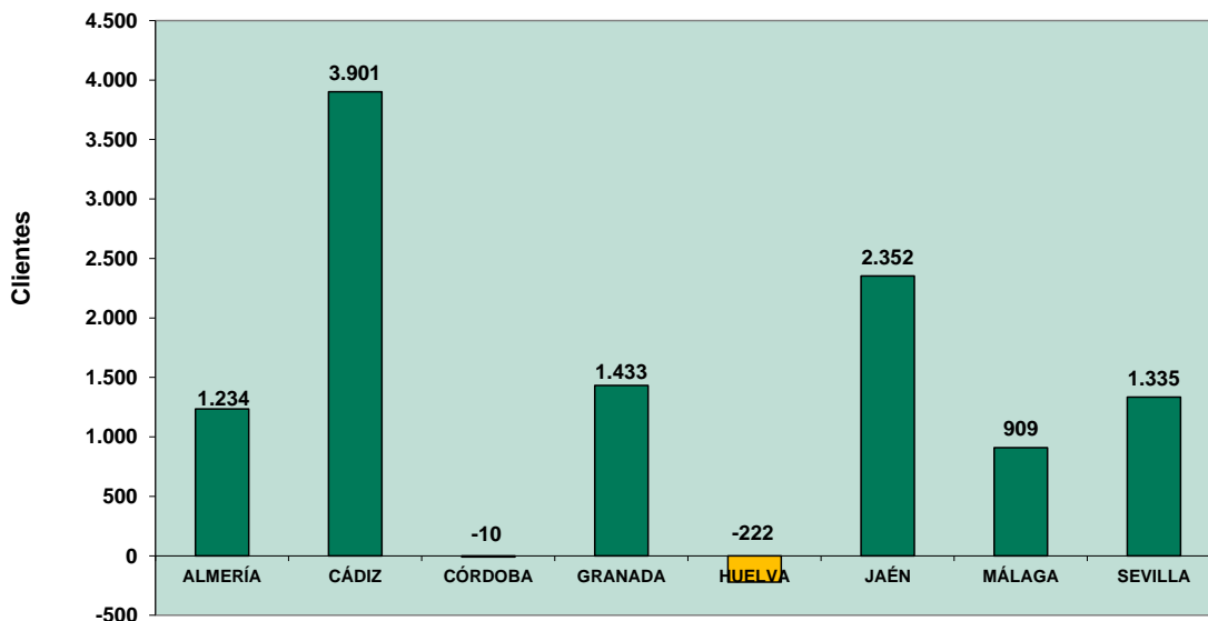
Figura 4. Crecimiento del número de clientes de gas natural en la Comunidad de Andalucía en el año 2017, por provincias.
