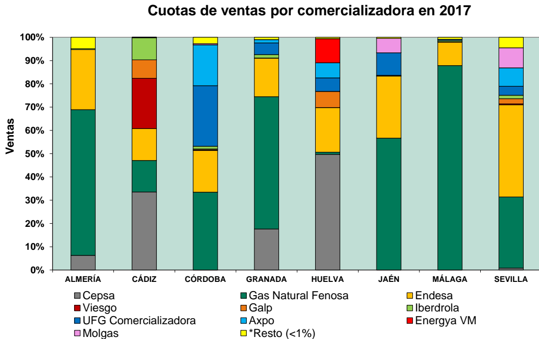
Figura 6. Cuotas de mercado por volumen de ventas de gas natural en la Comunidad de Andalucía en el año 2017, por grupo comercializador.
