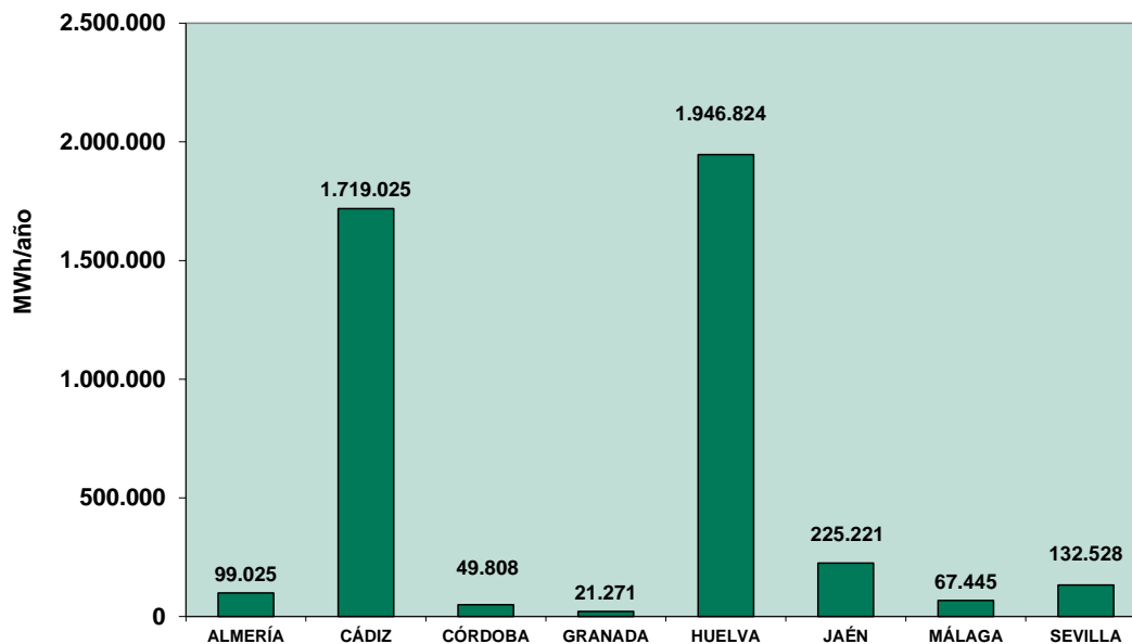
Figura 2. Variación del consumo de gas natural en la Comunidad de Andalucía en el año 2017, por provincias.
