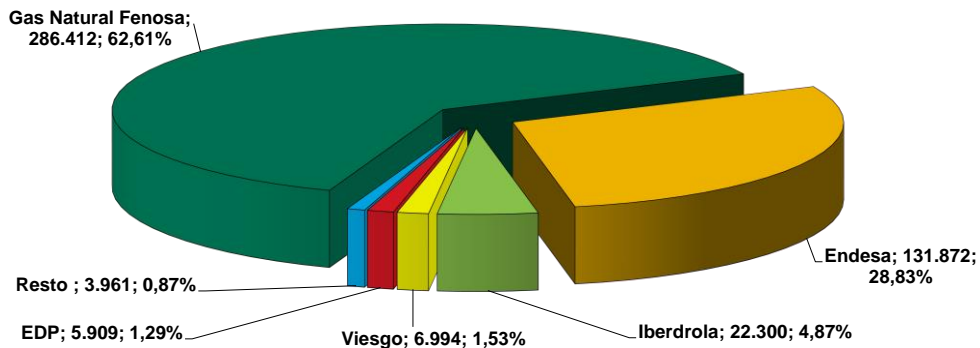
Figura 7. Cuotas de clientes de gas natural en la Comunidad de Andalucía en el año 2017, por comercializadora
