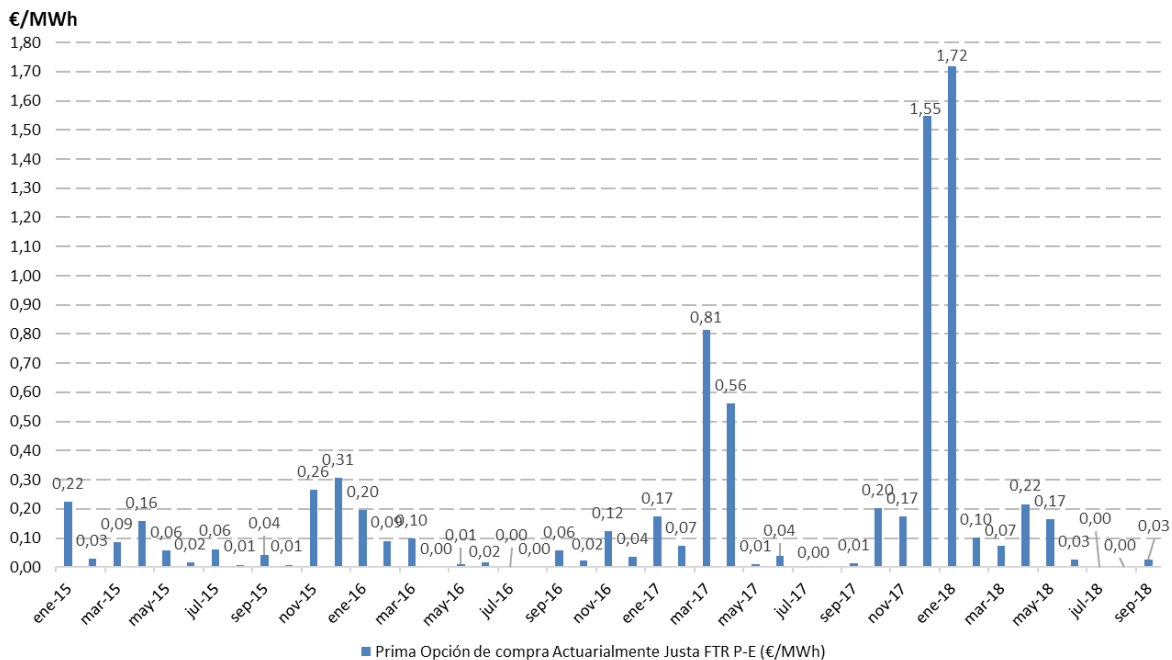
Gráfico 3. Referencias de precios medios del mercado spot ( P_P - P_E ) cuando P_P > P_E
