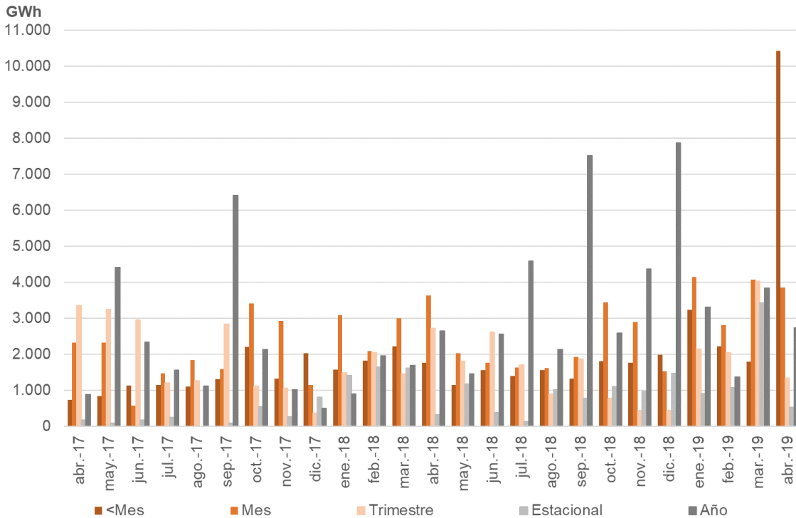
Gráfico 6. Volumen mensual de negociación (en GWh) en los mercados organizados y en el mercado OTC intermediado, por horizonte de entrega.
