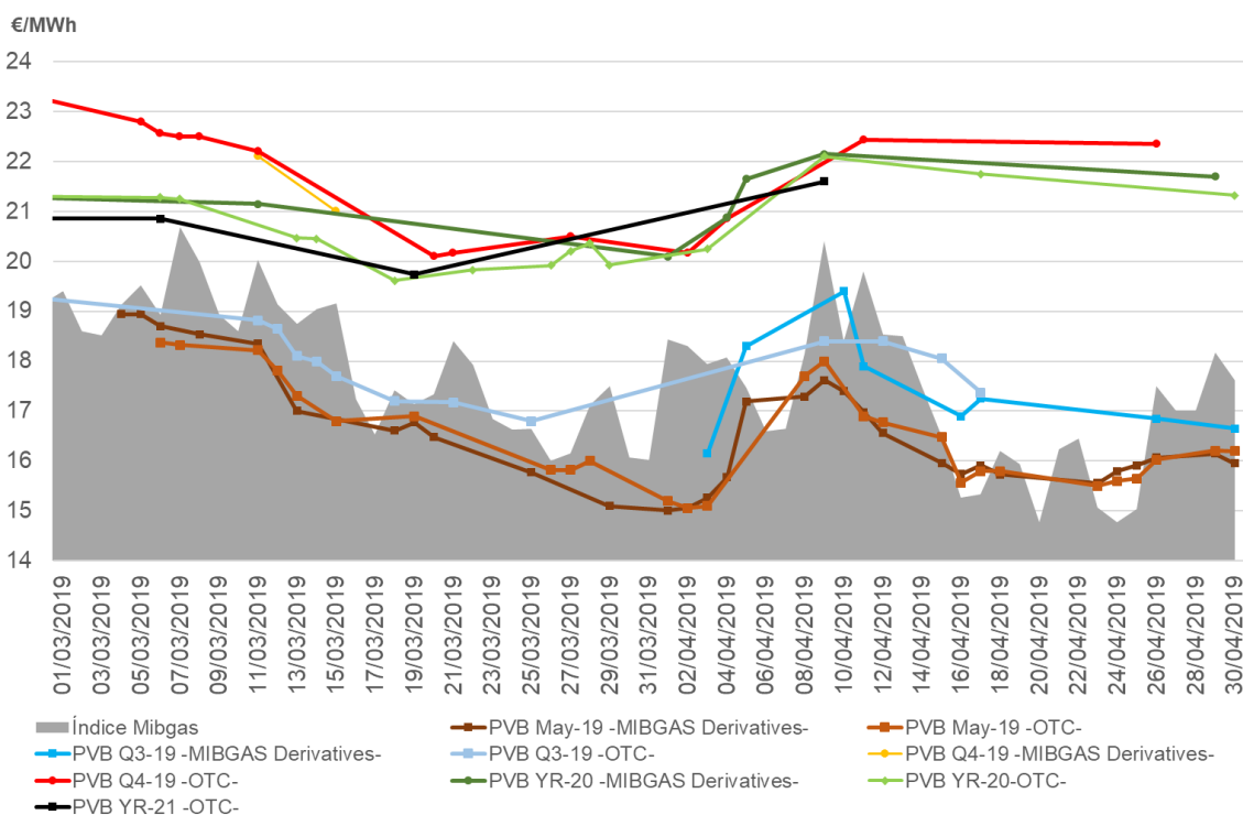
Gráfico 9. Evolución del índice MIBGAS-ES y de los precios a plazo de gas de los contratos de compraventa de gas con entrega igual o superior al mes, en PVB-ES, en MIBGAS, en MIBGAS Derivatives y en el mercado OTC intermediado. Del 1 de marzo al 30 de abril de 2019
