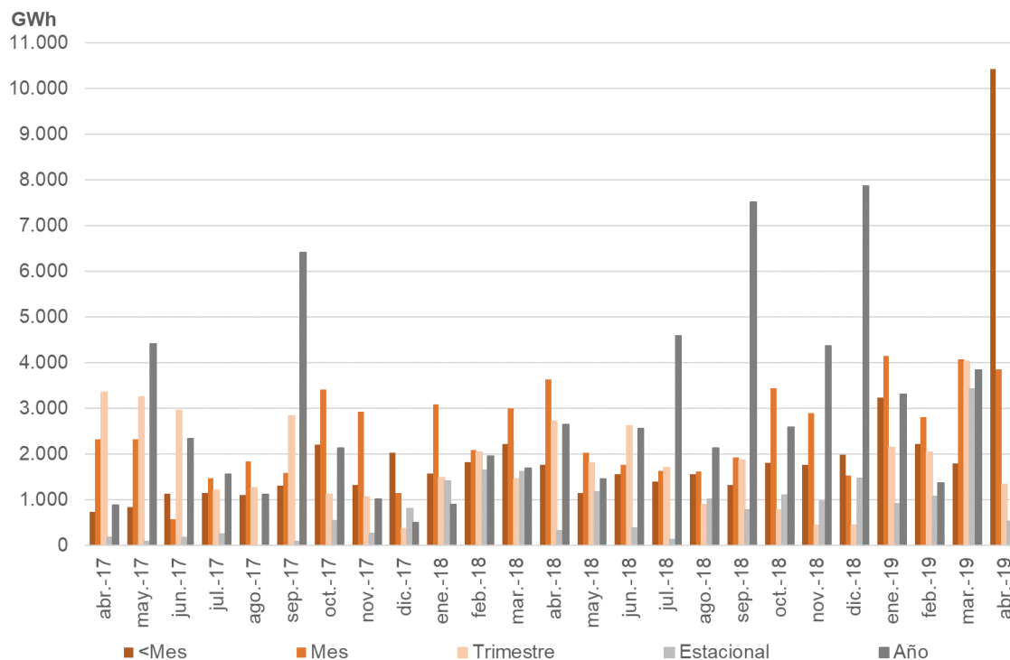
Gráfico 6. Volumen mensual de negociación (en GWh) en los mercados organizados y en el mercado OTC intermediado, por horizonte de entrega.
