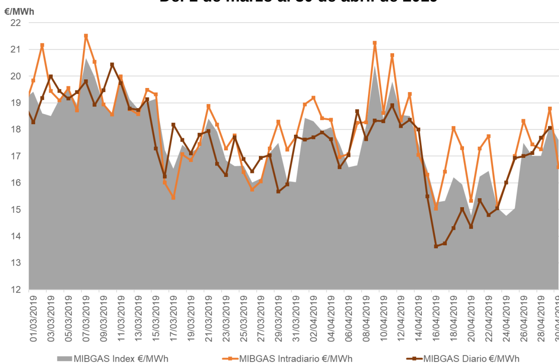
Gráfico 10. Evolución del índice MIBGAS-ES y de los precios a plazo de gas de los contratos de compraventa intradiario y diario correspondientes al día de gas que está siendo calculado, con entrega en el PVB-ES, negociado en MIBGAS. Del 1 de marzo al 30 de abril de 2019
