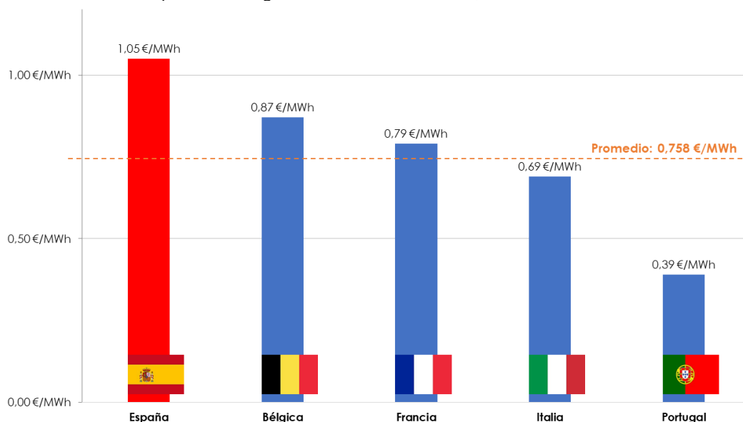
Gráfica 11: Coste total de descarga de un buque de 140.000 m³ de GNL, almacenamiento en planta y regasificación uniforme durante 10 días
