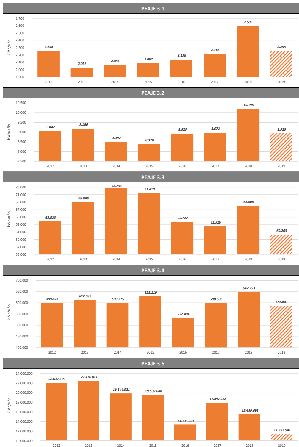
Gráfico I.2. Tamaños medios por peaje de acceso y tipo de consumidor registrado entre 2012 y 2018 y previstos para 2019 de los suministros de los suministros abastecidos desde plantas satélite
