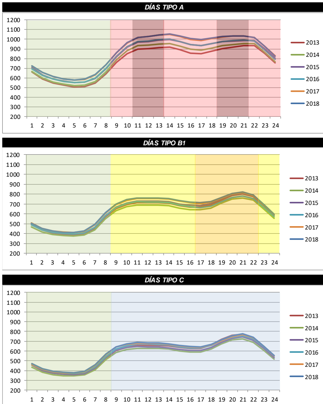
Gráfico II. 19. Potencia media horaria (MW) demandada por tipo de día según el calendario de la Orden ITC/2794/2007. Subsistema balear. Años 2013-2018
