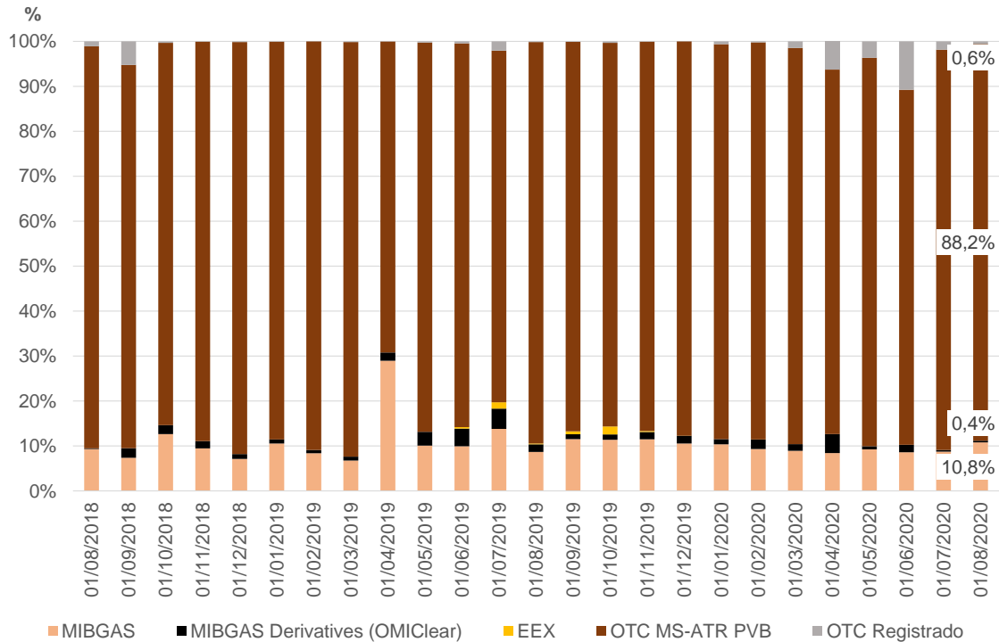
Gráfico 2. Volumen mensual negociado (en %) en los mercados organizados y en el mercado OTC (MS-ATR y registrados en cámaras). De agosto de 2018 a agosto de 2020
