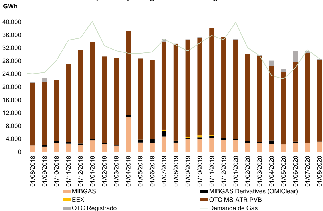
Gráfico 1. Volumen mensual negociado (en GWh) en los mercados organizados y en el mercado OTC (MS-ATR y registrados en cámaras) y demanda de gas natural (en GWh). De agosto de 2018 a agosto de 2020
