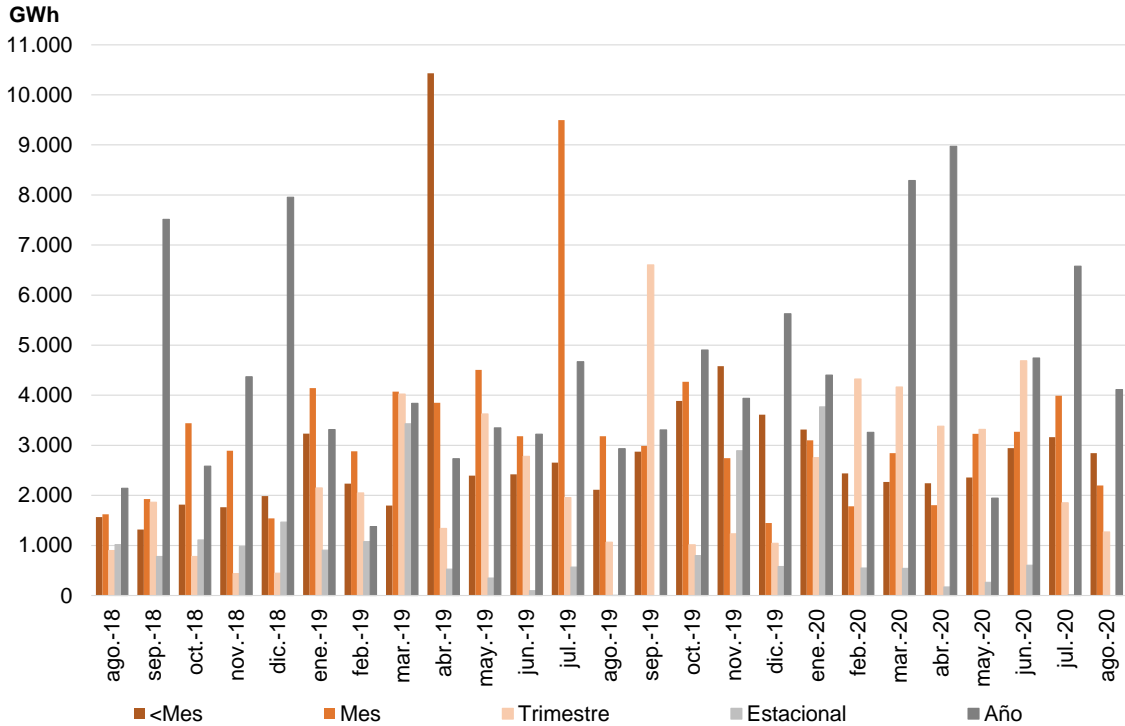
Gráfico 6. Volumen mensual de negociación (en GWh) en los mercados organizados y en el mercado OTC intermediado, por horizonte de entrega. De agosto de 2018 a agosto de 2020
