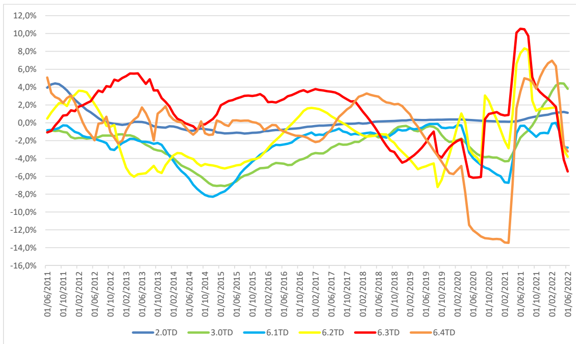
Gráfico I.4. Tasa de variación anual media de 12 meses de la potencia facturada por nivel de tensión
